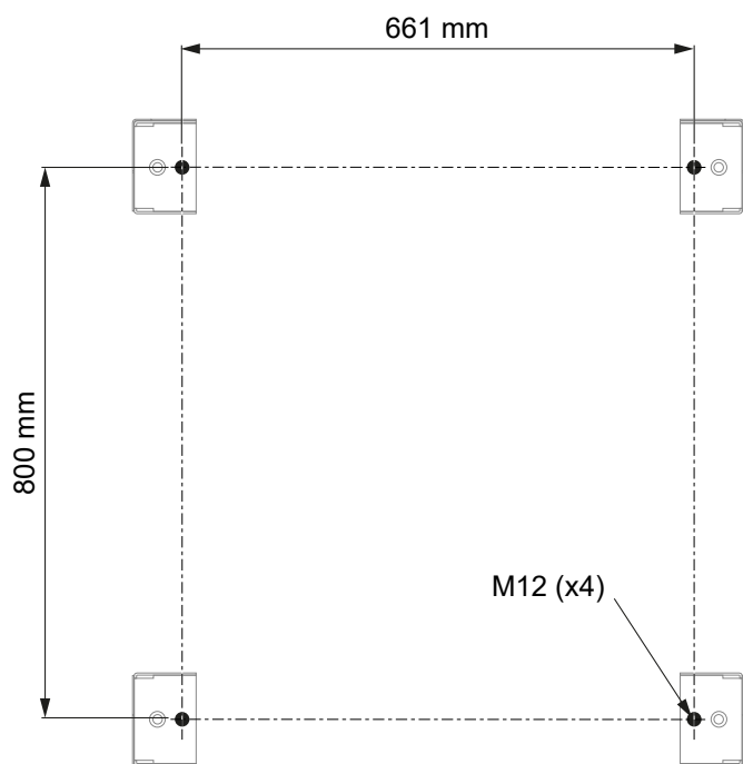
Installazione standard dell'UPS
