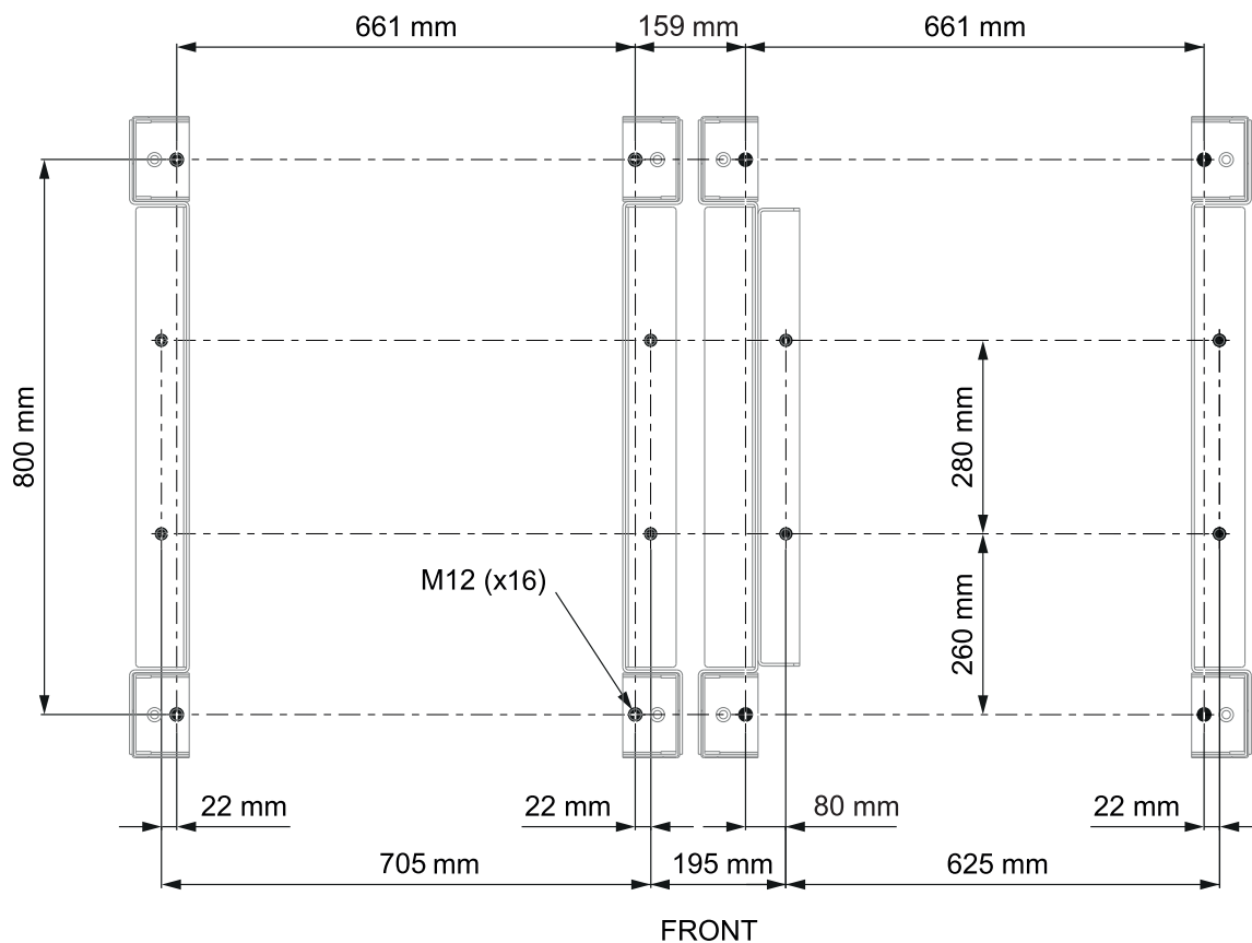
Installazione dell'UPS parallela per aree sismiche di Zona 4
