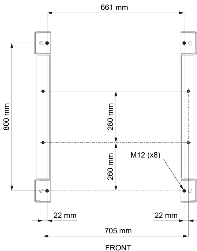
Installazione dell'UPS per aree sismiche di Zona 4
