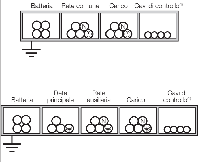
Installazione corretta
