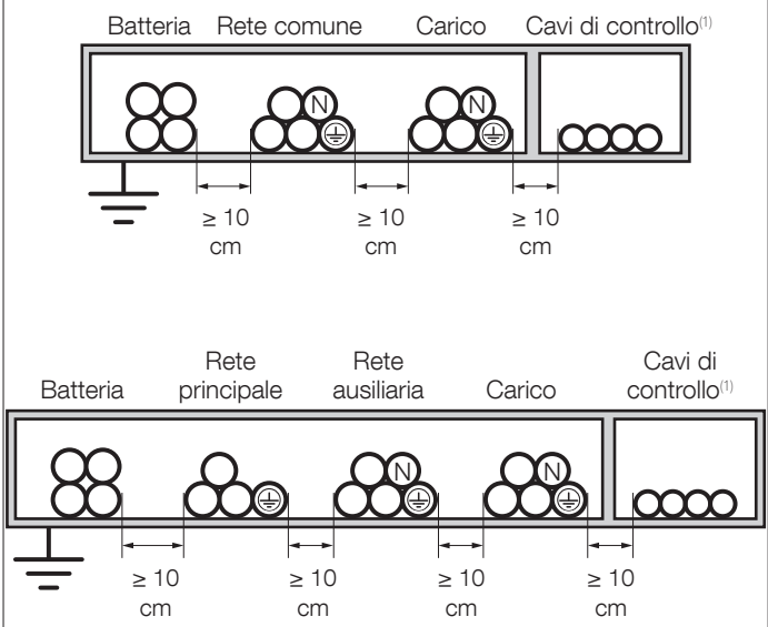
Installazione accettabile
