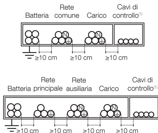
Installazione accettabile
