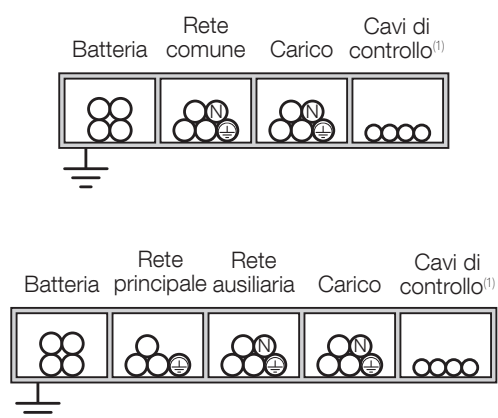
Installazione corretta
