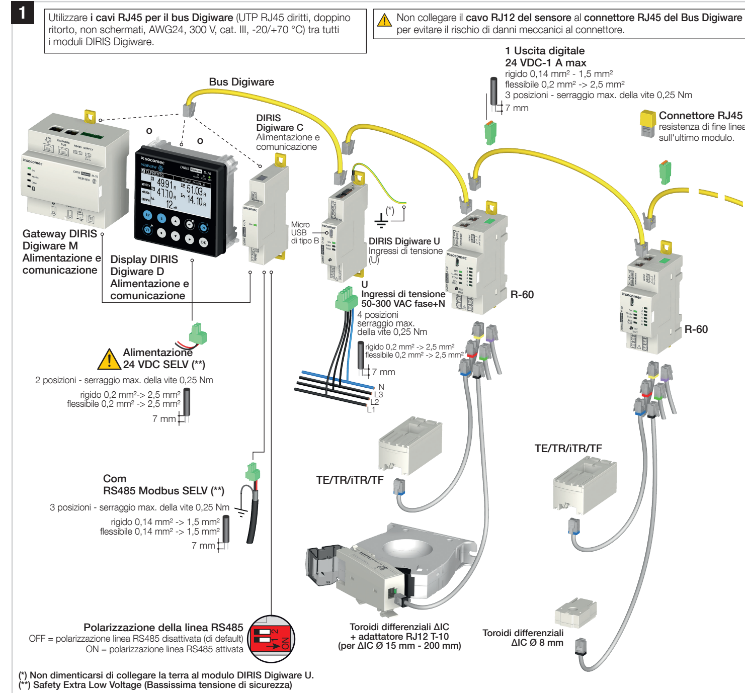
Dispositivo di monitoraggio della corrente residua DIRIS Digiware R-60 4829 0114
