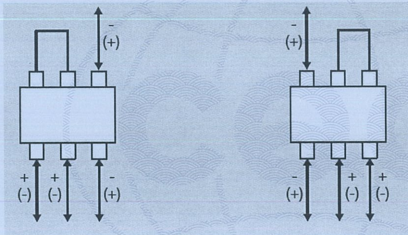
直流接线图
