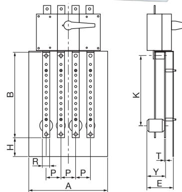
Ripartitore con connessione a mezzo capicorda, protezione frontale contro i contatti accidentali (apparecchio di sezionamento non fornito).
